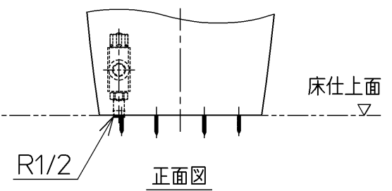
床給水仕様の場合
